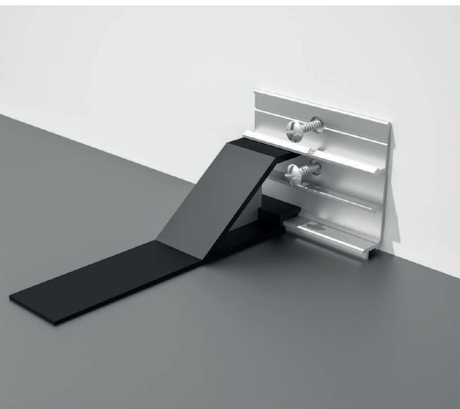
Particolare dello strumento utilizzato per posizionare in modo adeguato le guide per fissaggio battiscopa
