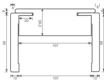
Particolare TELAI0 con FOGLIO BUSSOLA
