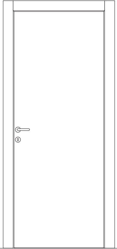
Telaio con coprifilo standard da 105 mm a 130 mm Frame with standard architrave from 105 to 130mm
