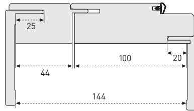
Telaio con ringrosso fino a 180 mm Frame with reinforcement up to 180mm
