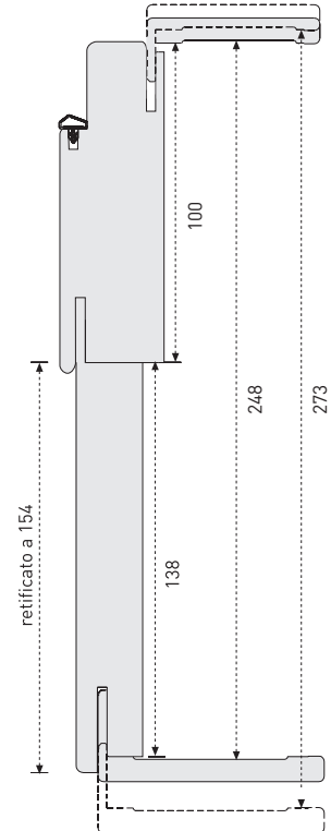
Telaio con foglio bussola fino a 273 mm Frame with socket sheet up to 273mm
