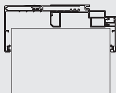
Telaio muro fino a 210 mm Wall frame wall up to 210 mm
