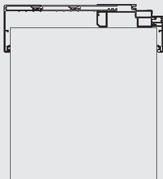
Telaio muro fino a 280 mm Wall frame wall up to 280 mm
